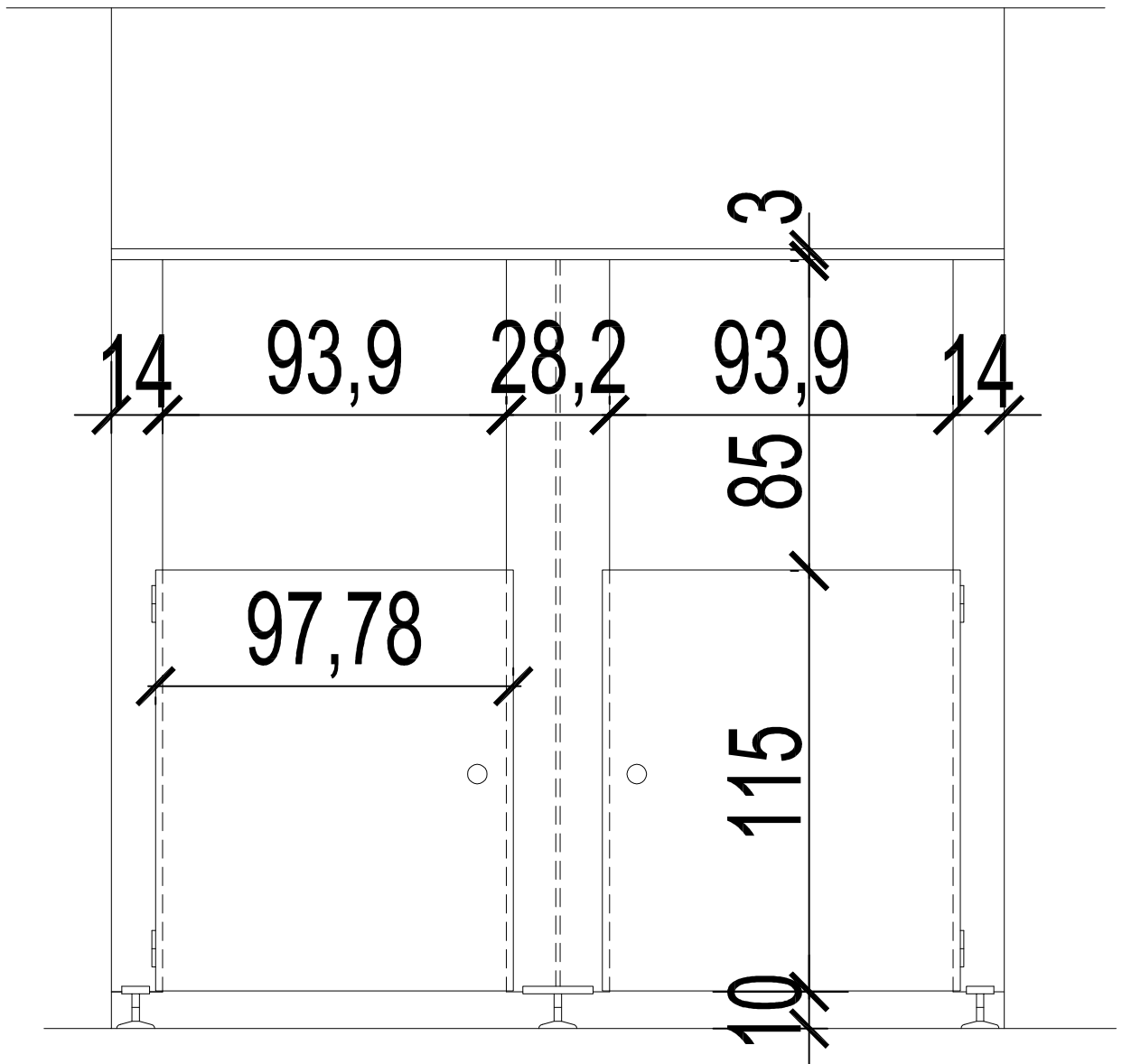
WIDOK NA ŚCIANKĘ CZOŁOWĄ
