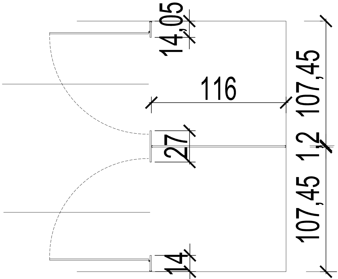
RZUT PRZEGRÓD WC
